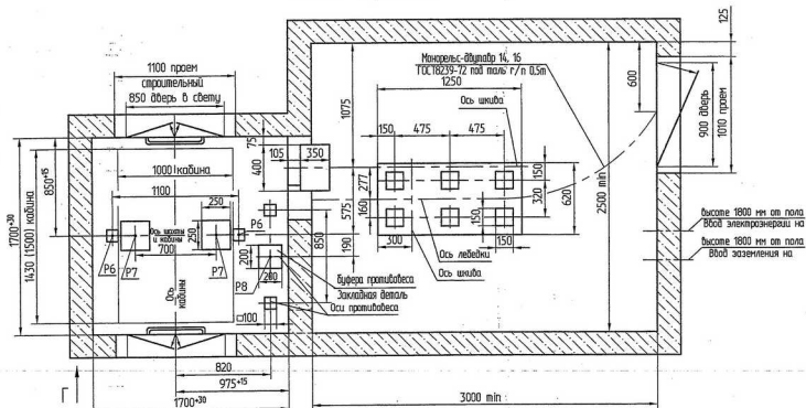
В-В (1) Вариант 2
