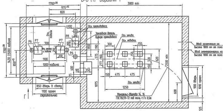
План шахты и машинного помещения
