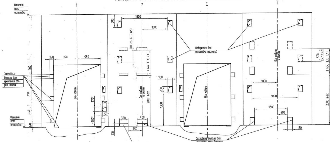
План шахты
