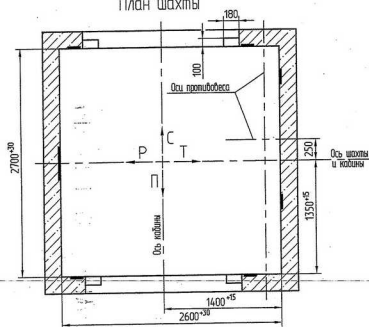
План шахты
